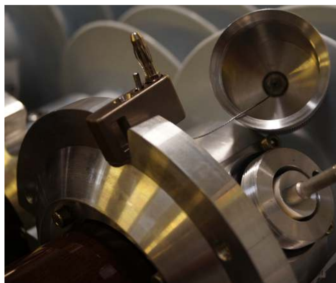
Рис. 7б измерительный вывод со снятым колпаком
